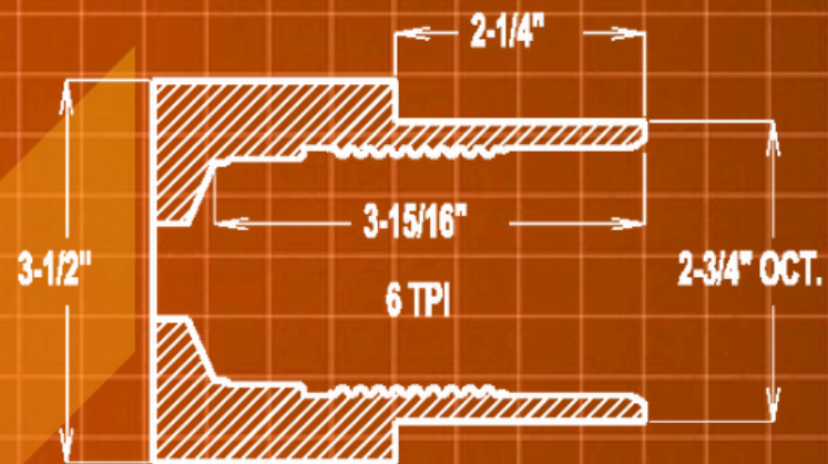
2.25-6 EZ2 BOX
