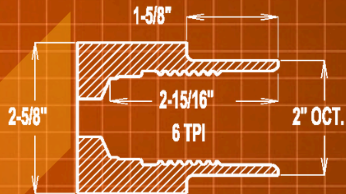
1.63-6 EZ2 BOX
