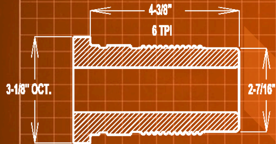
2.63-6 EZ2 PIN
