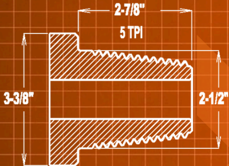
2-3/8" REG API PIN
