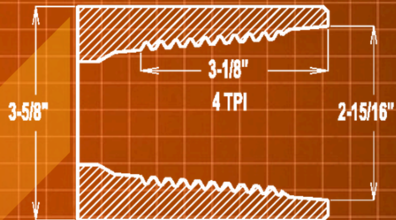
2-3/8" I F BOX
