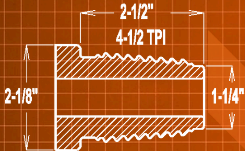
1.9" FS1 PIN #250
