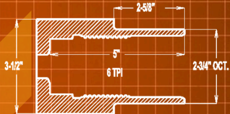
2.25-6 EZ3 BOX
