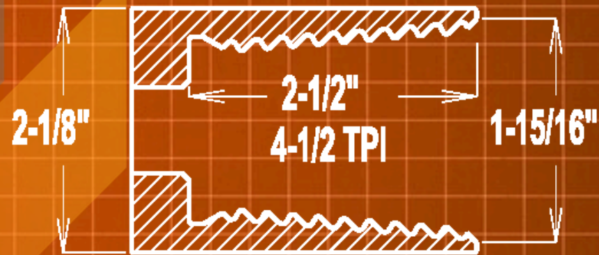
1.9" FS1 BOX #250
