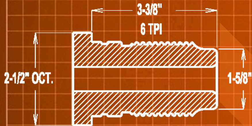
2.0-6 EZ2 PIN
