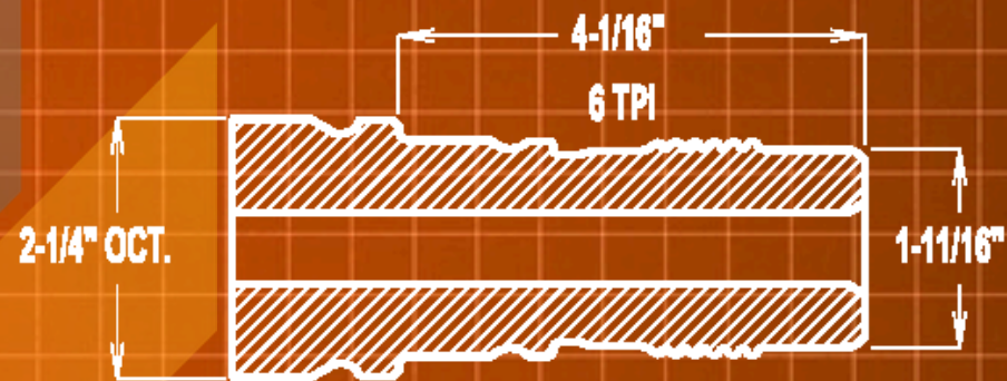
1.88-6 EZ3 PIN
