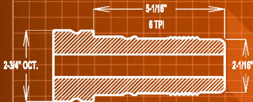
2.25-6 EZ3 PIN
