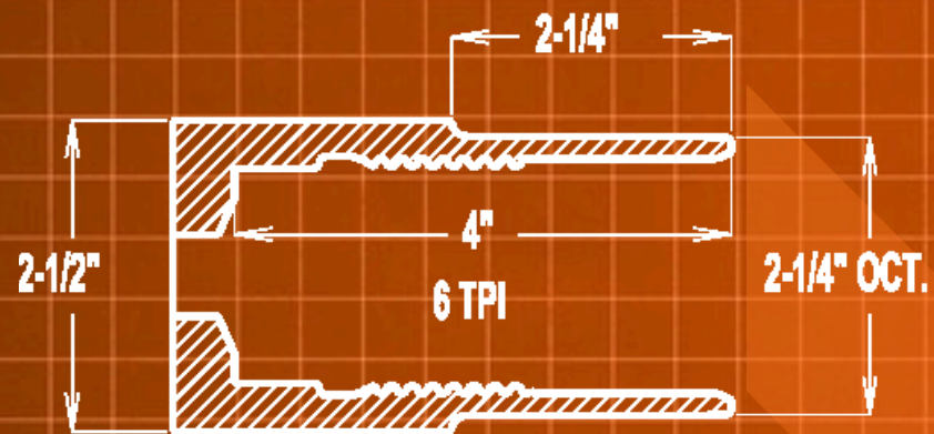
1.88-6 EZ3 BOX
