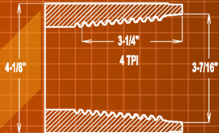
3.25-4 BOX
