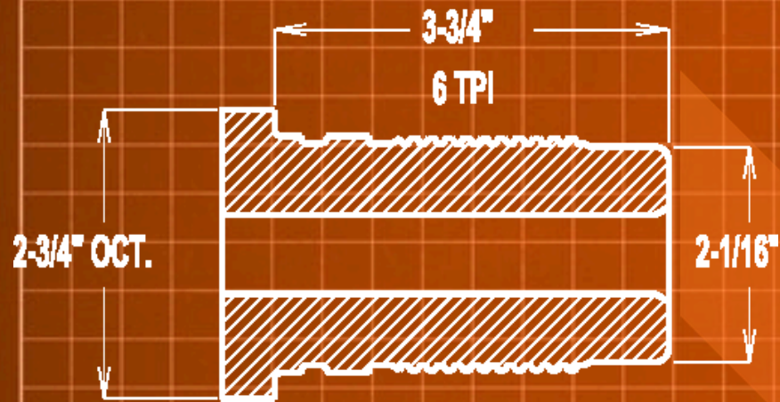
2.25-6 EZ2 PIN
