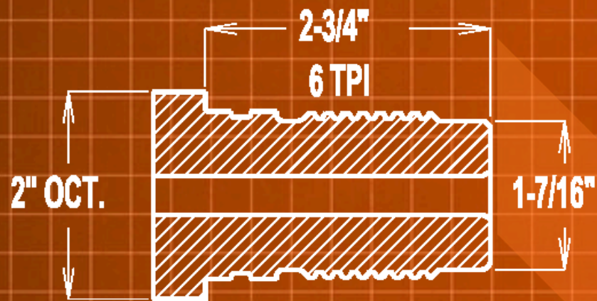
1.63-6 EZ2 PIN
