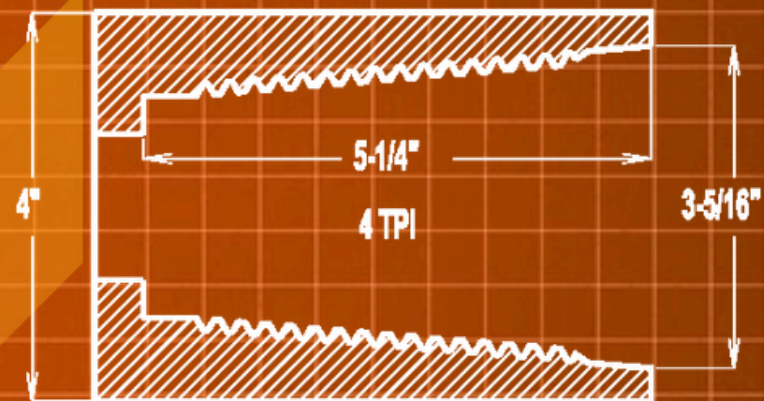
3.27-4 BOX
